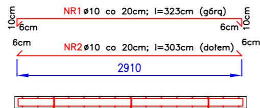
PŁYTA ŻELBETOWA "SU2.9"
