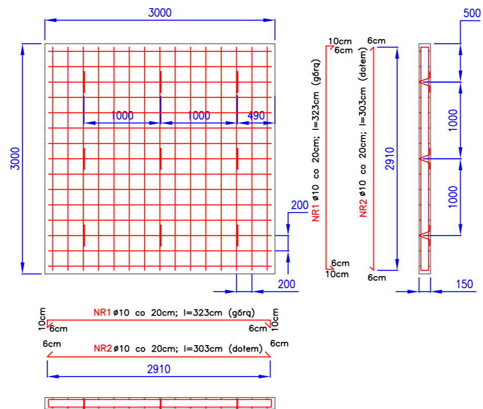
PŁYTA ŻELBETOWA "SU2.9"
