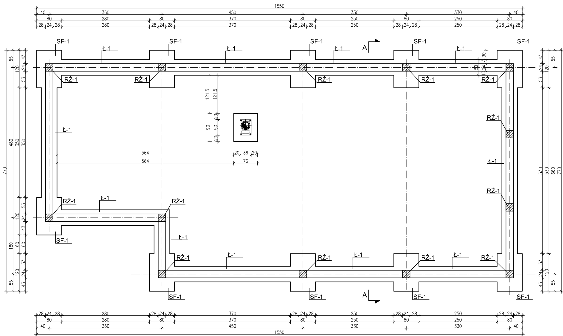
RZUT FUNDAMENTÓW 1:50
