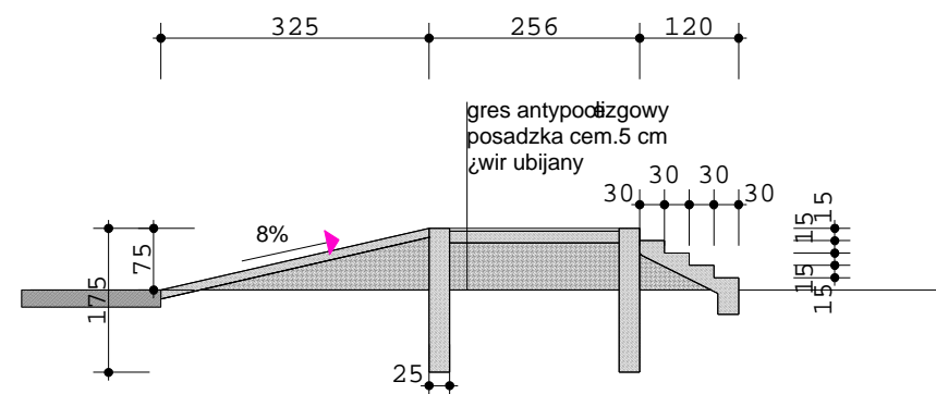
PRZEKRÓJ 5a-5a
